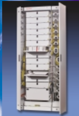
FIST-GR2 Стойка повышенной емкости с оптическими распределителями и системой организации пассивных компонентов сети. Комплексные решения для оптических кросс всех типов
